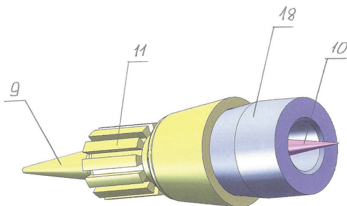
Рисунок 7. Интегральный интерфейс устройства для смешивания, гомогенизации и активирования жидких смесей, жидкостей и сжатых газов
