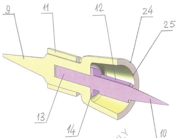
Рисунок 10. Осевое сечение интегрального интерфейса устройства
